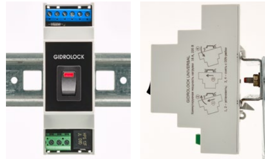
Фото 1, 2. Блок управления системы GIDROLOCK UNIVERSAL, установленный на DIN-рейку.
