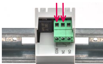
Фото 5. Подключение электрического насоса к блоку управления.
